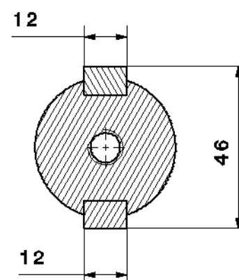
SchnittB-B Maßstab: 2:3
