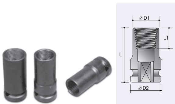
Deep
