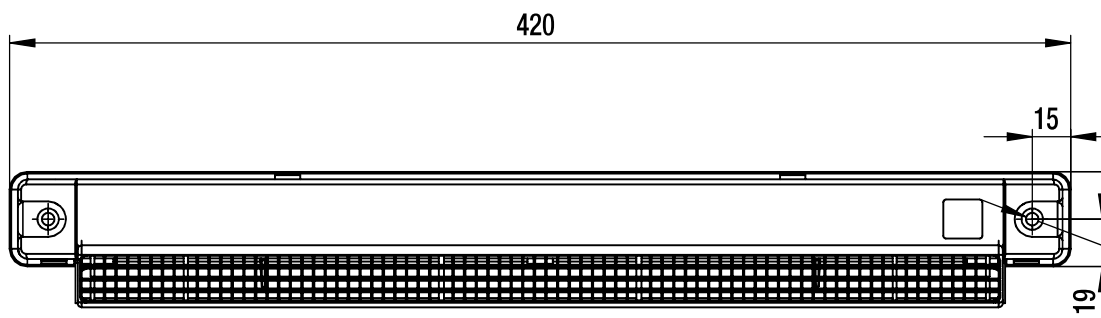
WHAI 02 - Frontansicht
