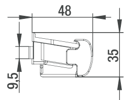
Seitenansicht
